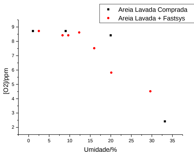
Figura 8 – Quantidade de oxigênio obtida com sensor
