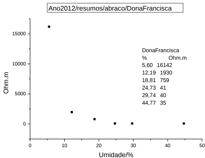
Figura 4 – Resistividade em função da umidade para Dona Chica
