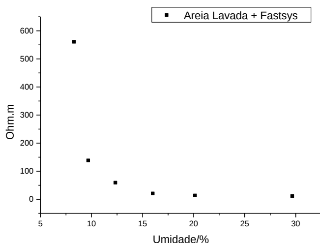
Figura 6 – Variação da resistividade para areia lavada com aditivo
