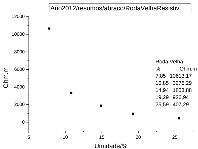
Figura 3 – Resistividade em função da umidade para Roda Velha
