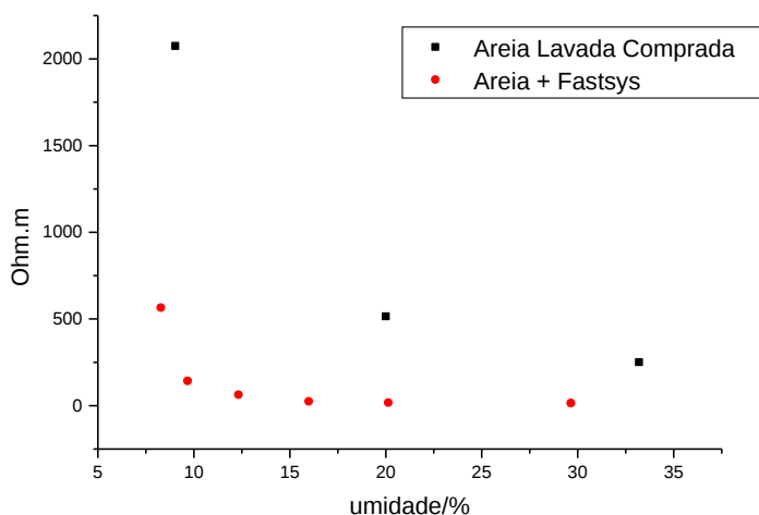
Figura 7 – Variação da resistividade para amostras estudadas
