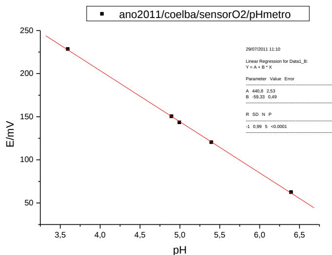
Figura 2 – Potencial medido no terminal 1 do sensor em relação ao pH
