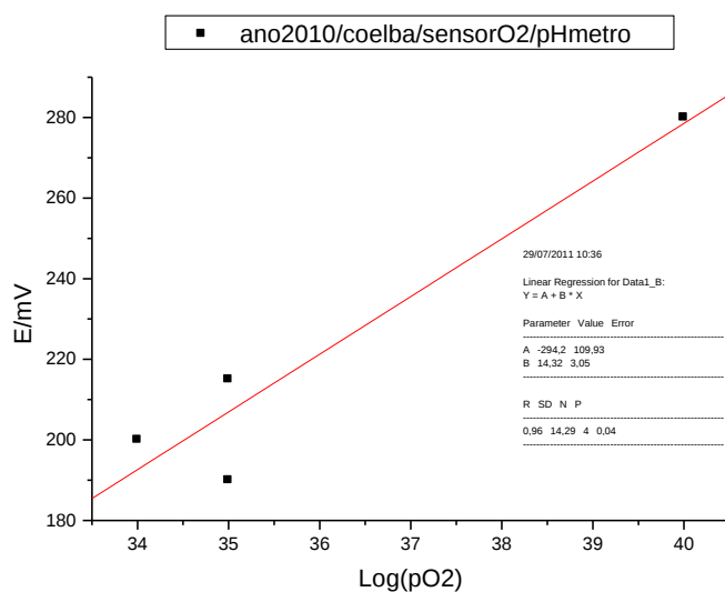
Figura 1 – Potencial do terminal 2 do sensor em relação ao \log p_{O_2}
